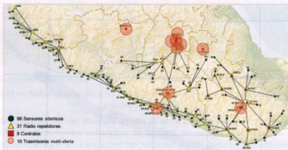
Figura 9. Sensores Sísmicos, Topología de enlaces y Difusión de Alerta del SASMEX®
