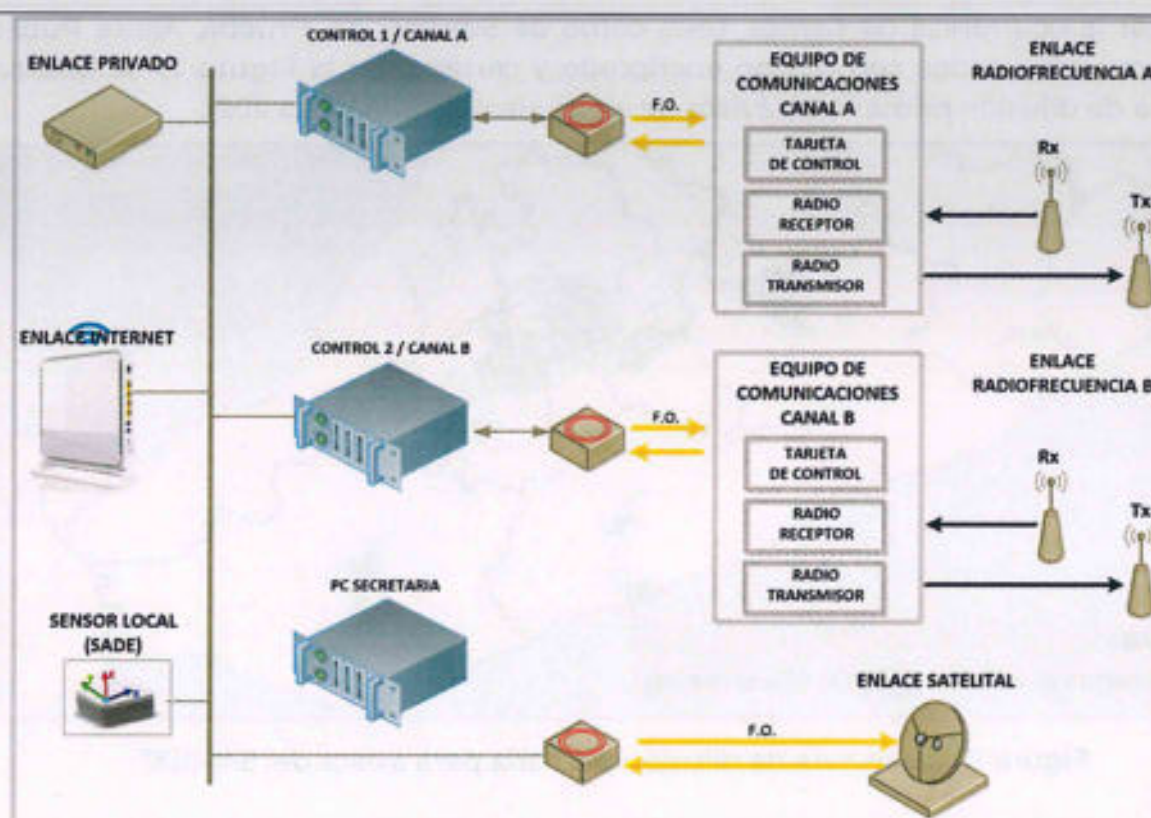
Figura 16. Diagrama a bloques de la EASAS.
