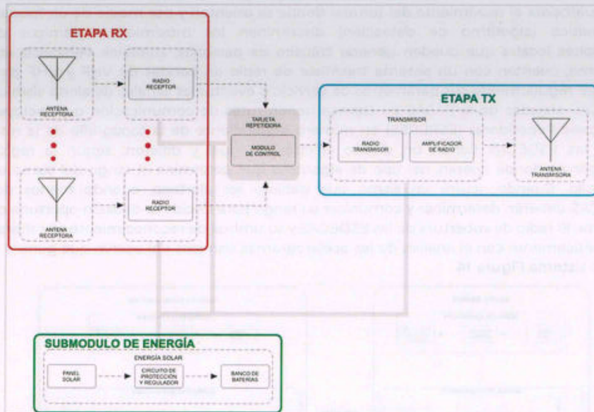
Figura 15. Diagrama a Bloques de la ESREPE.
