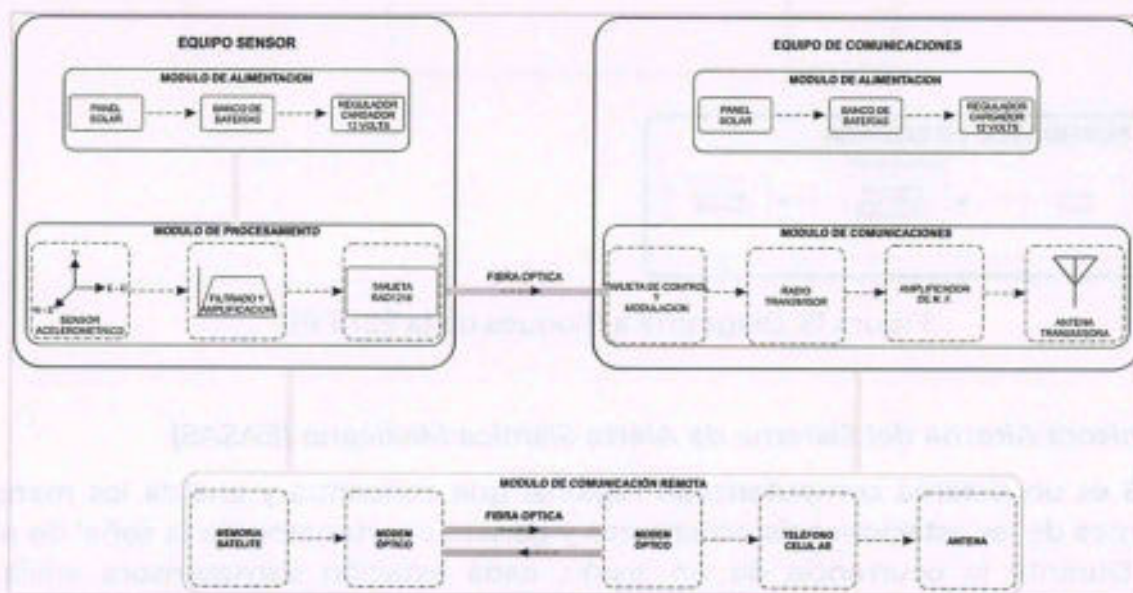
Figura 14. Diagrama a Bloques de la ESDECA.
