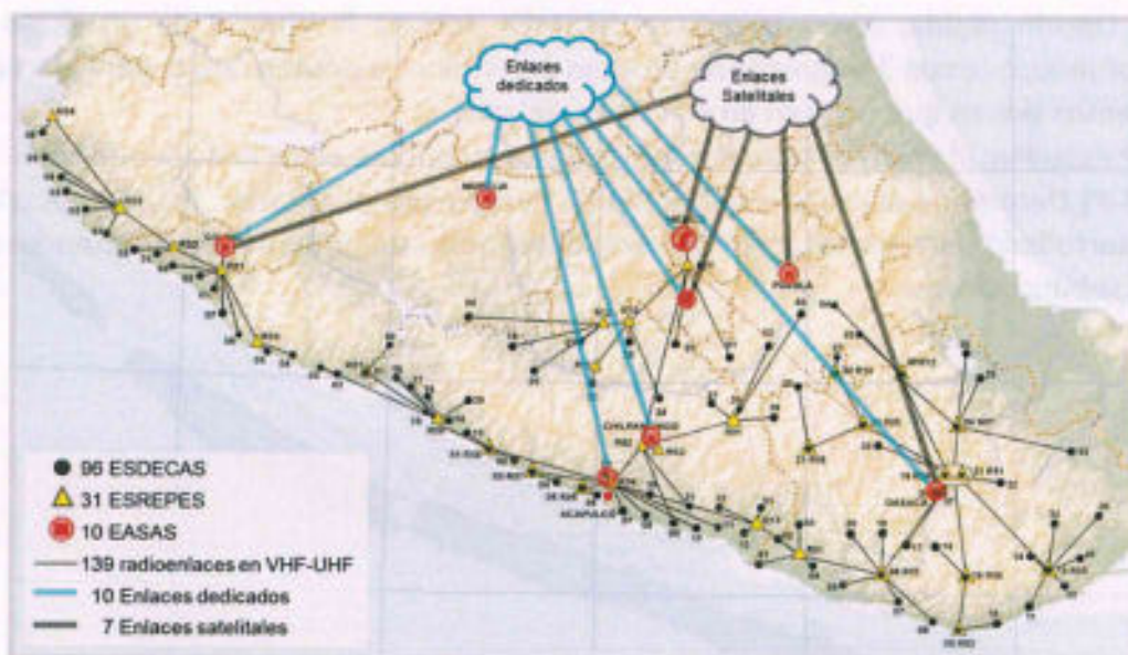
Figura 7. Sensores Sísmicos y Topología de enlaces del SASMEX®
