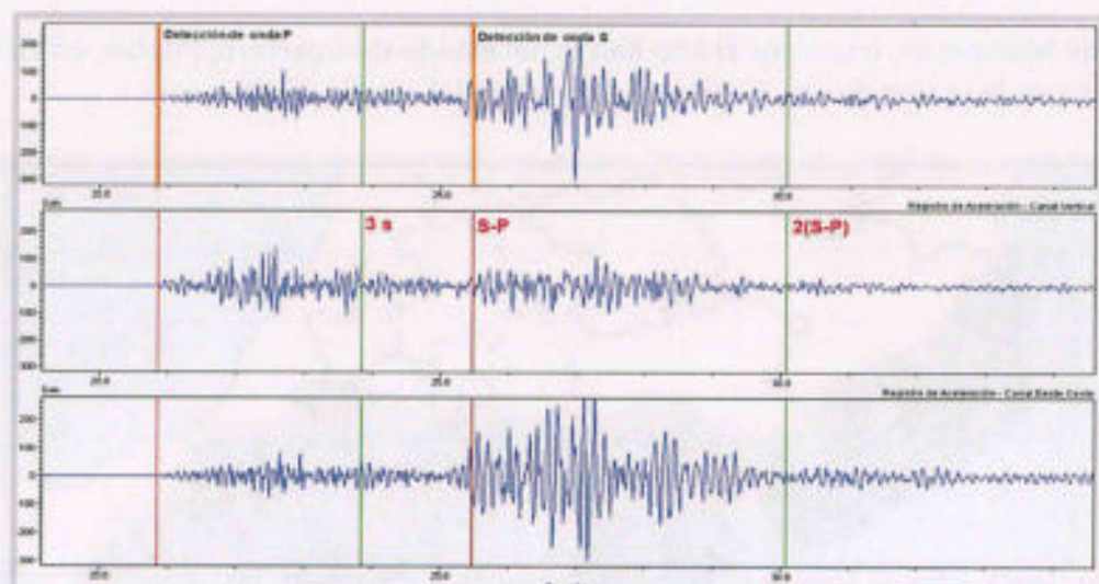
Figura 6. Algoritmos de detección del SASMEX®
