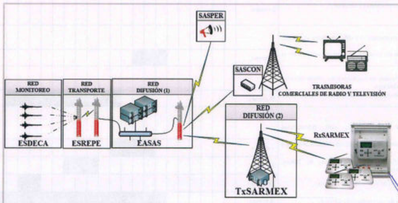
Figura 13. Diagrama de la infraestructura del SASMEX®.
