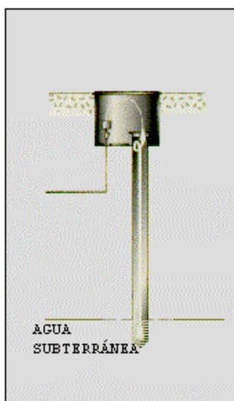
Figura 5.3.2 Pozo de observación para agua subterránea
