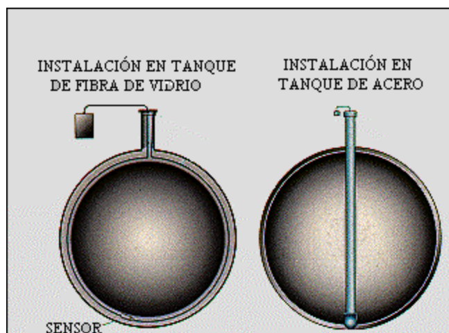
Figura 5.2.4 Sistema de monitoreo intersticial para detectar presencia de fugas en el interior del tanque o fuera de él
