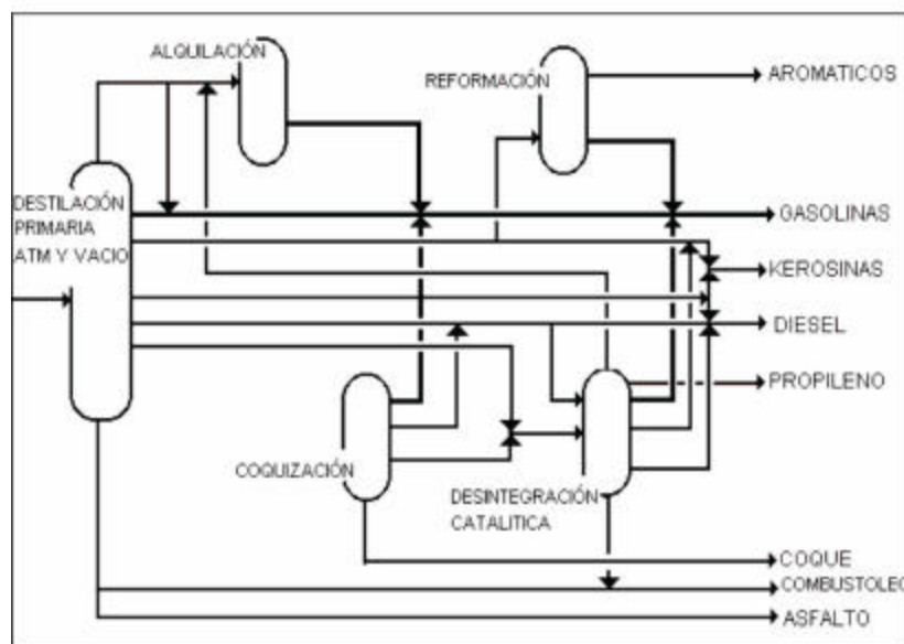
Diagrama 2.1 Proceso de Refinación Simplificado
