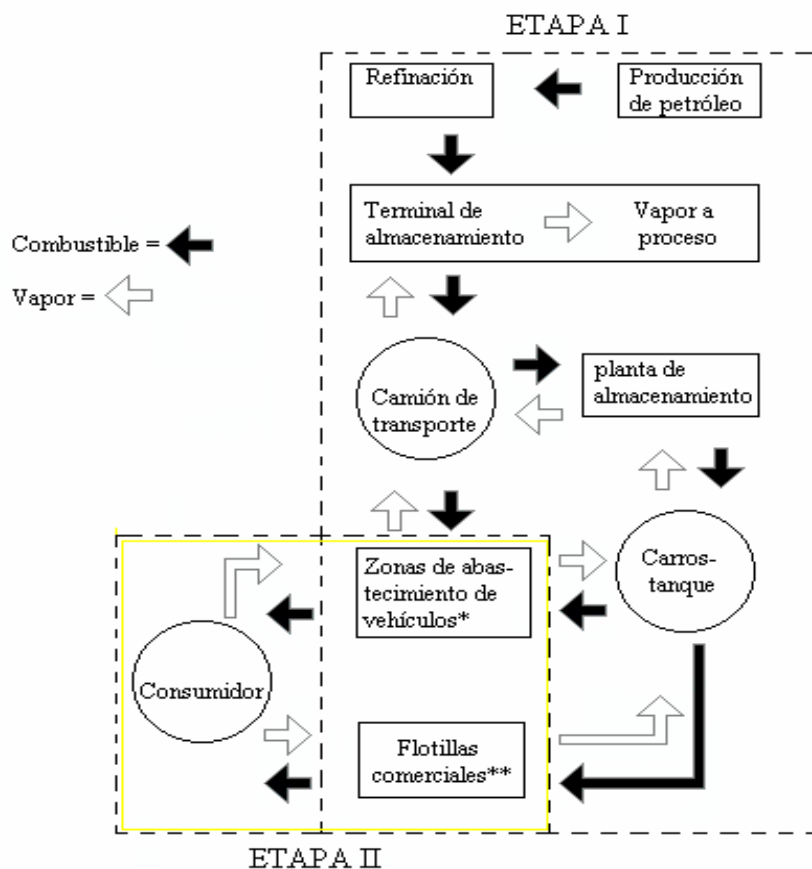
Figura 5.5 Control de emisiones durante la distribución que hacen los carros tanques y en las operaciones de abastecimiento a vehículos en estaciones de servicio
