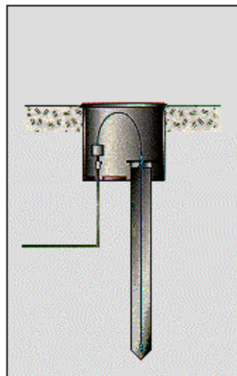
Figura 5.3.1 Sensor de pozo de vapor para monitoreo de hidrocarburo en suelos
