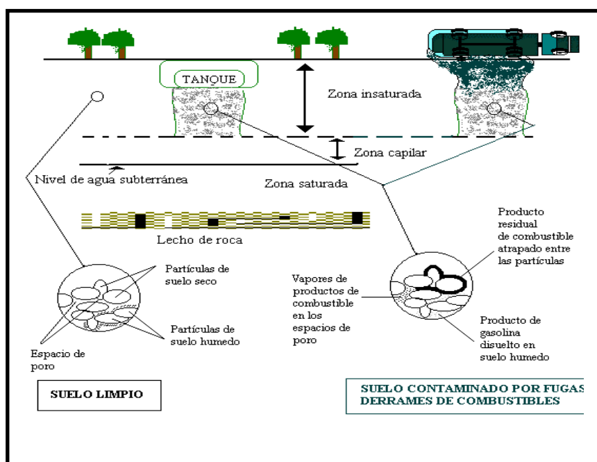
Figura 4.2 Representación de las tres fases diferentes en las cuales pueden ser encontrados los hidrocarburos en la zona insaturada
