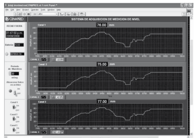
Pruebas realizadas con 3 sensores de nivel en la misma sección de medición
