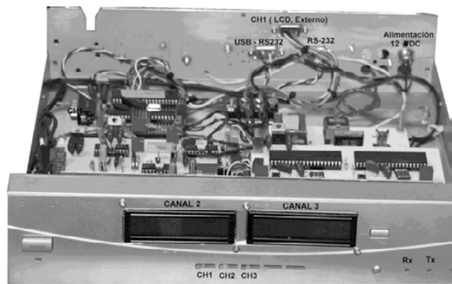
Módulo de pruebas del nuevo protocolo de estación de medición de nivel
