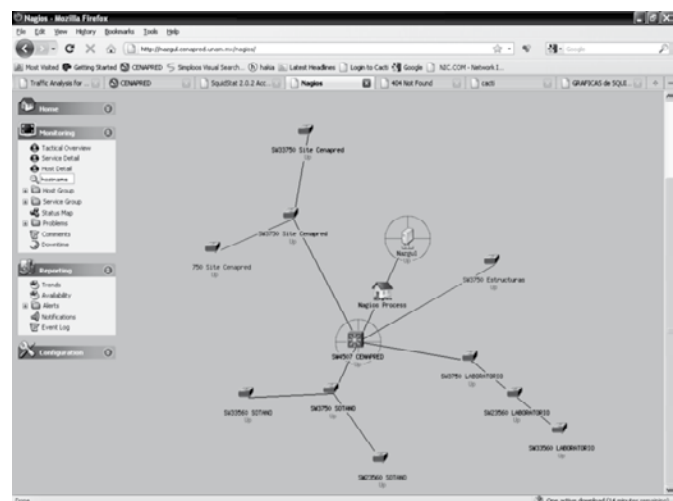
Interfaz Gráfica de Nagios
