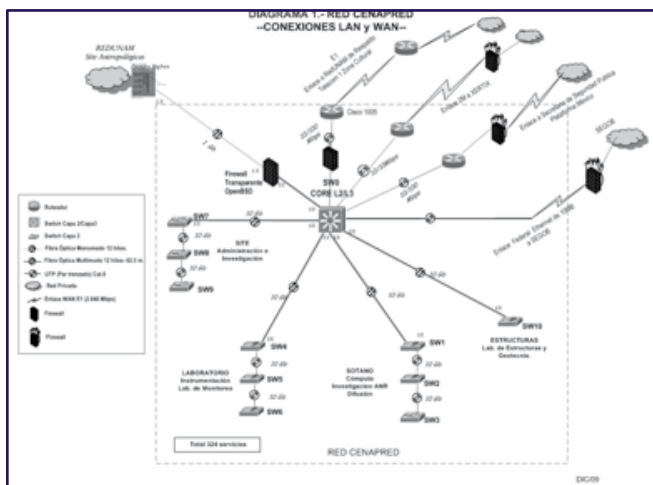
Diagrama de Red LAN y WAN.
