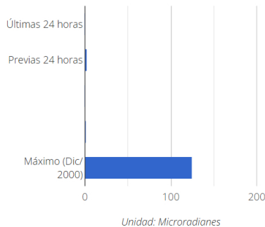
Deformación (Inclinómetros)
